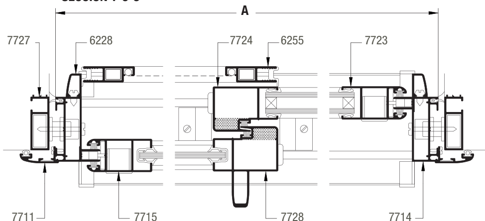
SECCION 1-6-3
