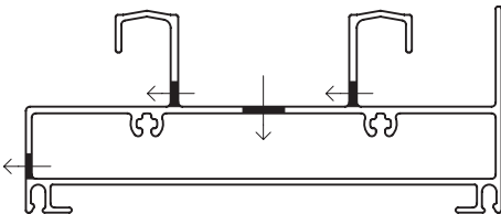
ESQUEMA DESAGÜES GUIA UMBRAL
